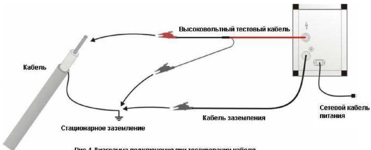
Рис.4 Диаграмма подключения при тестировании кабеля
